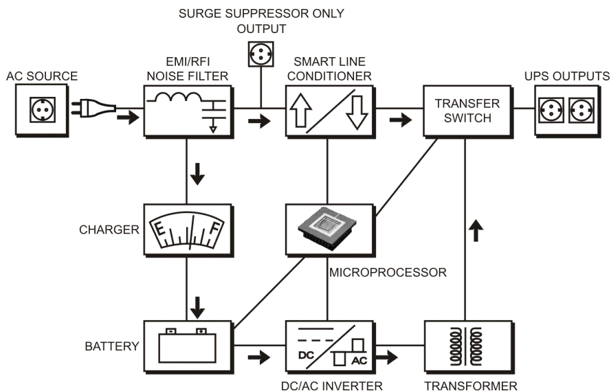
شکل ۱: ساختار داخلی یوپی‌اس‌های سری VENU
